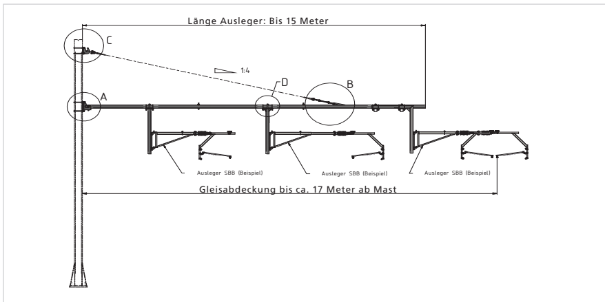
Maximale Auslegerlängen
