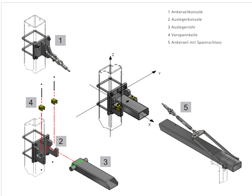
Einfache Befestigung am Mast dank patentiertem System
