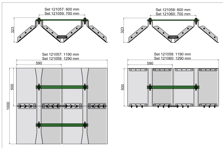
Aufbauschema: Basispaket, Ein- und Ausfahrmodul
