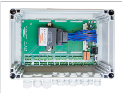
Weichensteuerung KUSCOI Artikel-Nr. C2513-02
